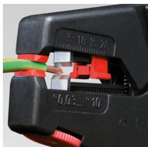
12 40 200: Прецизно сваляне на изолацията без повреждане на проводника
